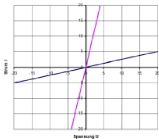
Strom / Spannungsdiagramm
