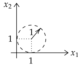
Abbildung 3: Epsilon-Umgebung
