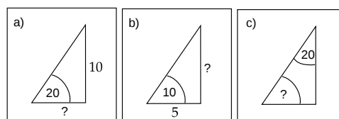
Abbildung 12: rechtwinklige Dreiecke
