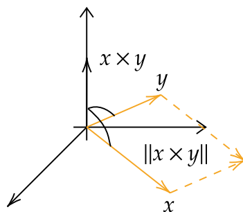
Abbildung 16: Kreuzprodukt
