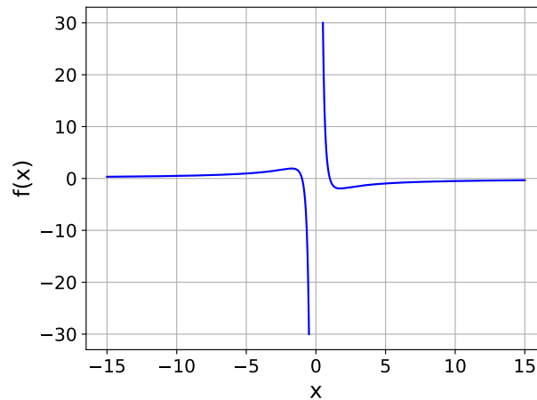
Abbildung 18: Kurvendiskussion
